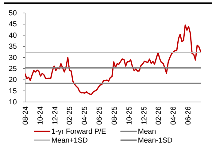
图 4: 前瞻市盈率
