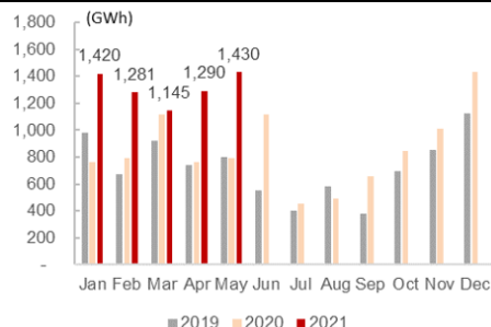
新天绿色能源之月度风电发电量
