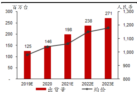
小米之智能手机出货量预测
